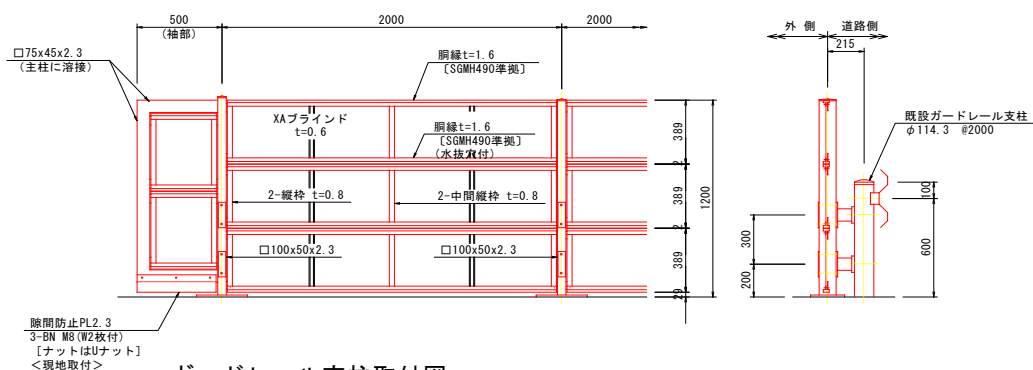
パネル取付図
